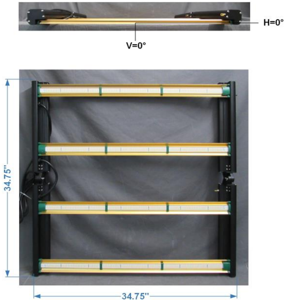
FIG. 1 LUMINAIRE
