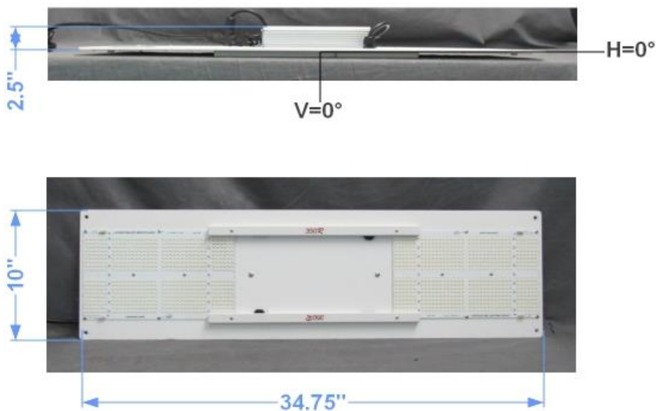
FIG. 1 LUMINAIRE
