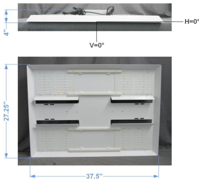
FIG. 1 LUMINAIRE
