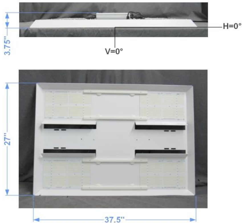
FIG. 1 LUMINAIRE
