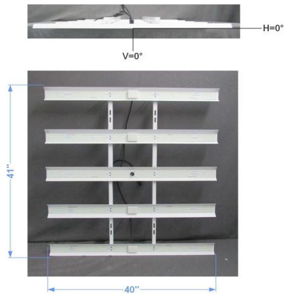
FIG. 1 LUMINAIRE
