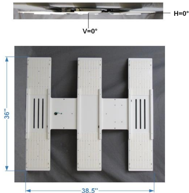
FIG. 1 LUMINAIRE
